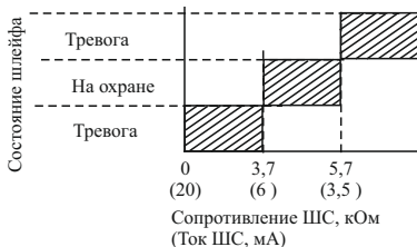
Рисунок 5 – Шлейф охранных извещателей (тип 6)
